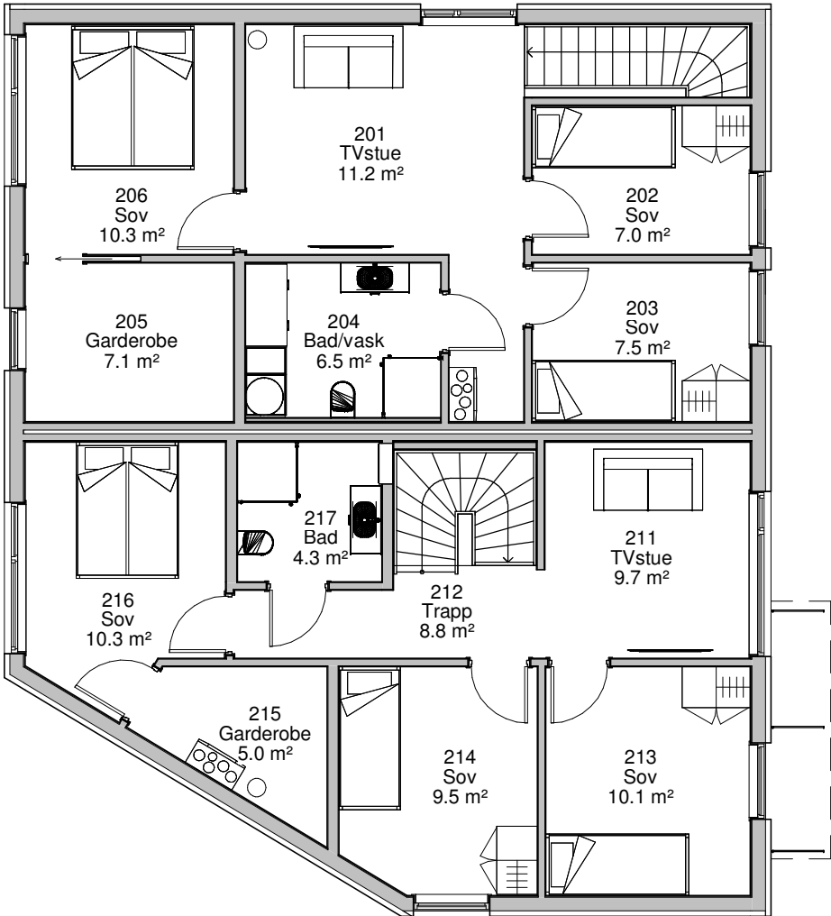
Plan 2-etg.
