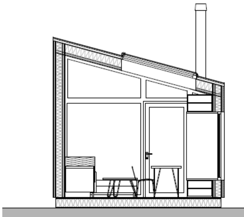
Snitt A4
