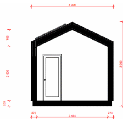
Snitt A1
