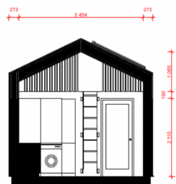
Snitt A3
