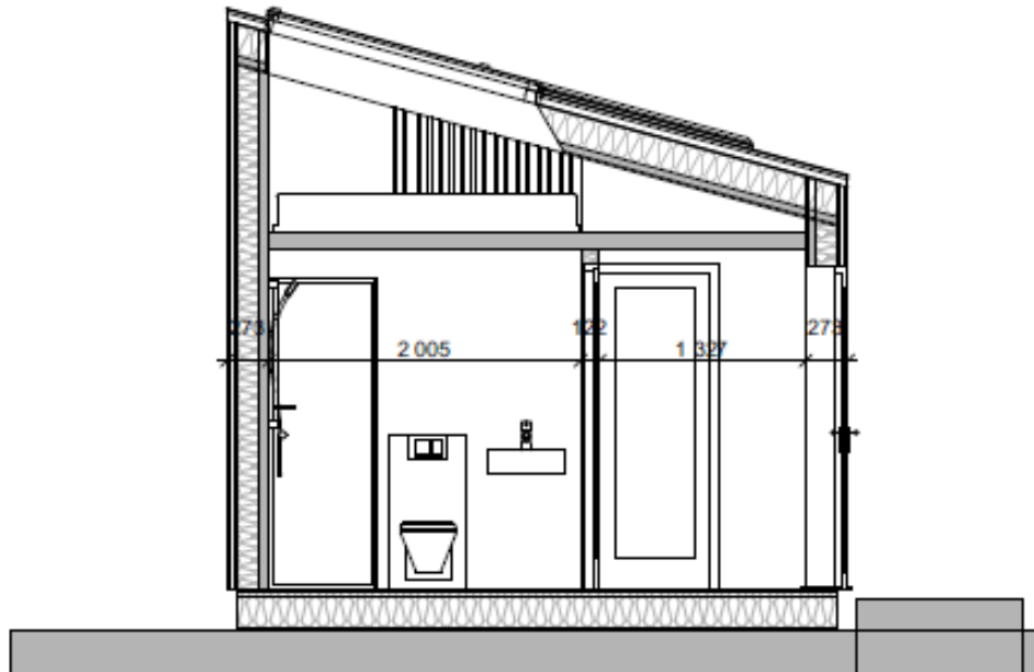
Snitt A2
