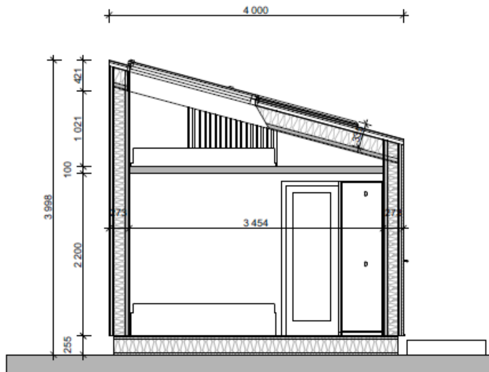
Snitt A1
