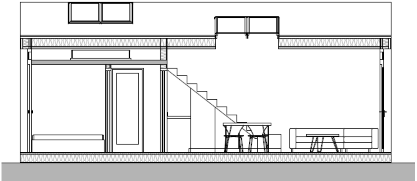
Snitt B2
