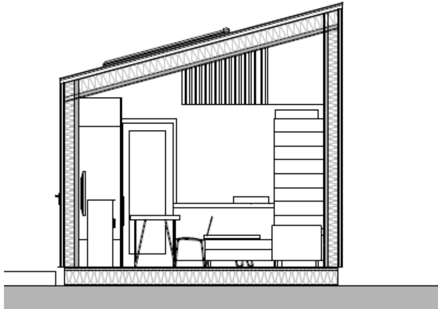
Snitt A5
