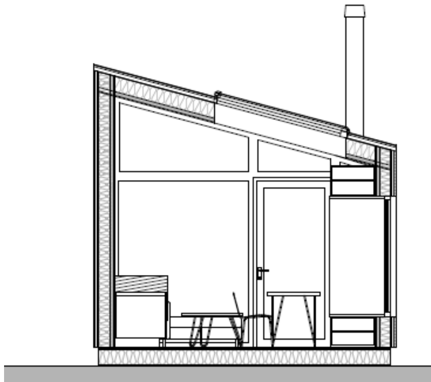
Snitt A4
