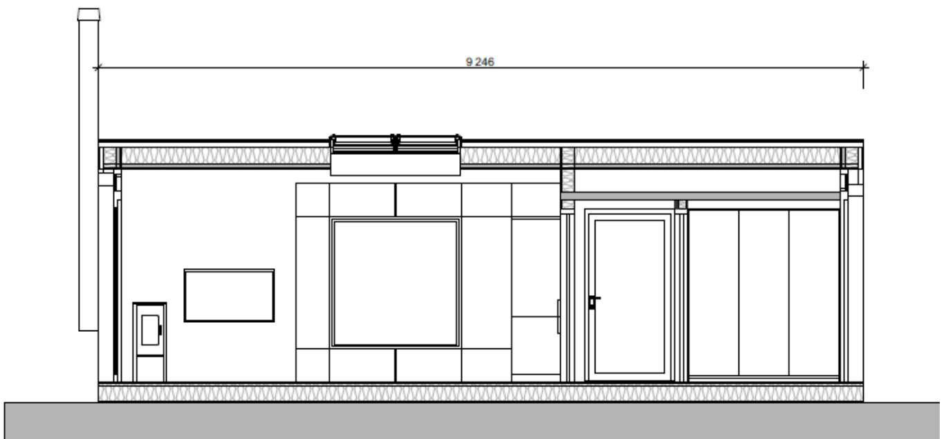
Snitt B1
